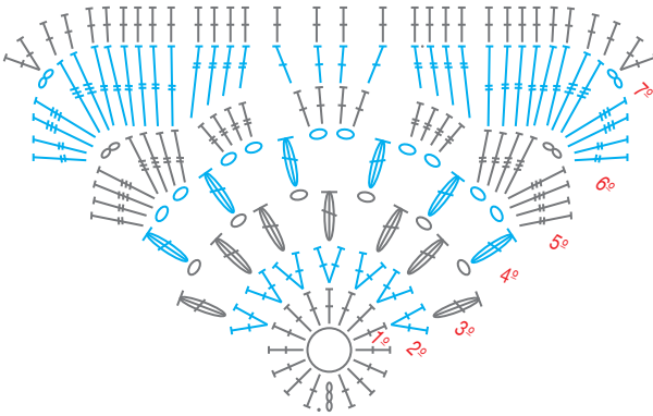
Diagrama N° 3 (borde superior del bolso)
