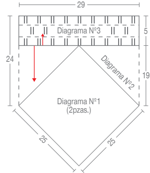
Diagrama N° 3 (borde superior del bolso)
